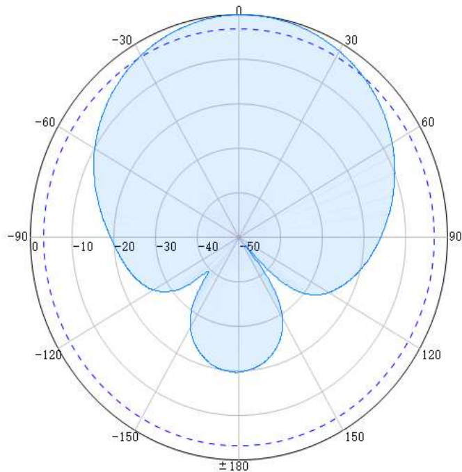
Horizontal (866MHz)
